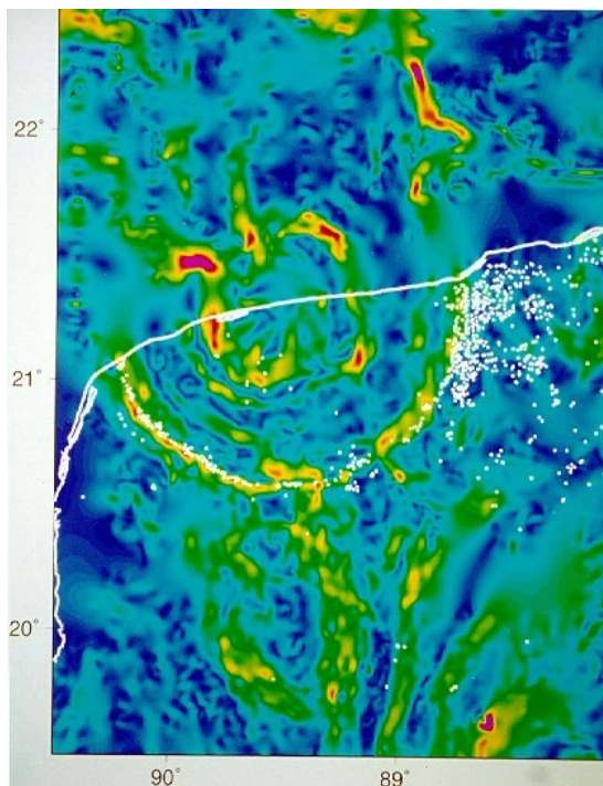
Image gravimétrique du cratère de Chicxulub. Le trait blanc représente la côte Nord de la péninsule du Yucatán (Mexique). Crédit : Geological Survey of Canada.
